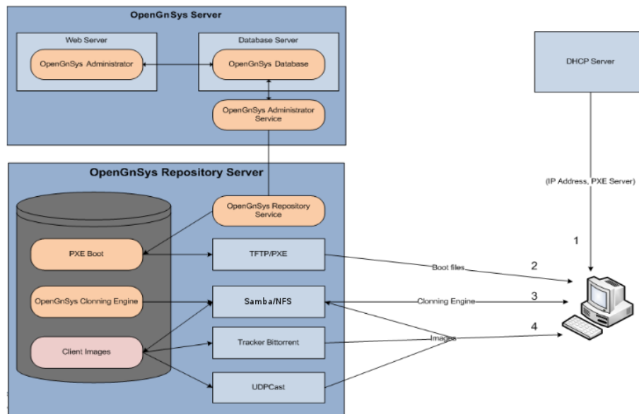
Arquitectura de componentes de OpenGnsys
